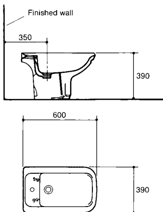
Astros Bidette D-0263/64
