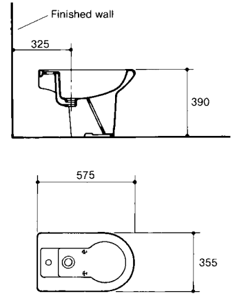
Calypso Bidette D-1877
