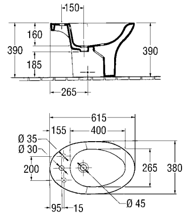
Presqu'île Bidette D-1K48/3K48
