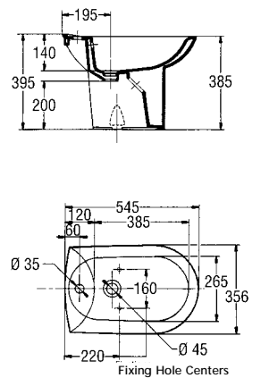
Odeon Bidette D-1K38
