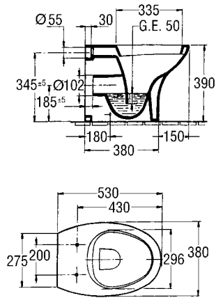
Presqu'île Wall-Faced Pan D-6K60
