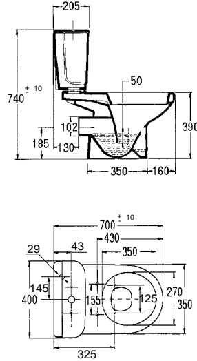
Calypso P-Trap Toilet D-1892/1952
