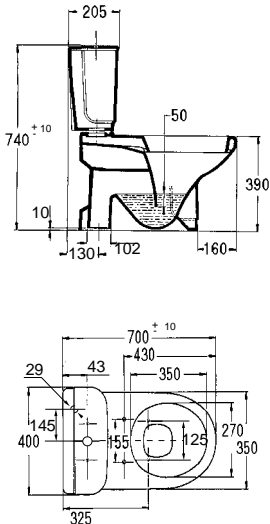
Calypso® Toilet D-1815/1952
