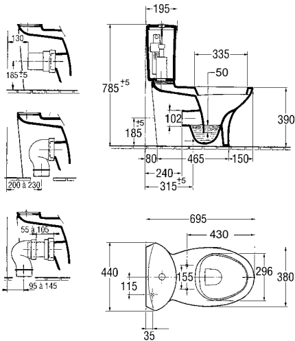
Presqu'île Toilet D-6K72/8K25
