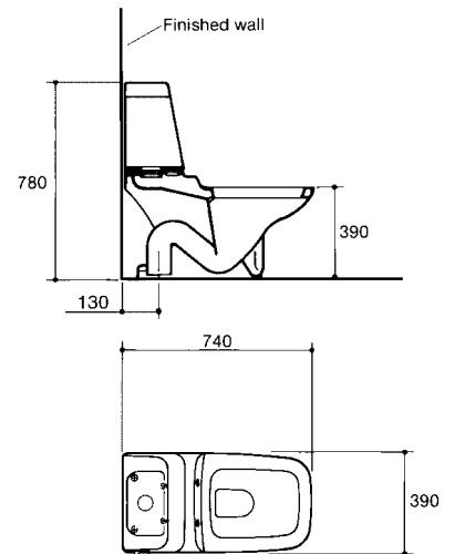
Astros® Toilet D-0470
